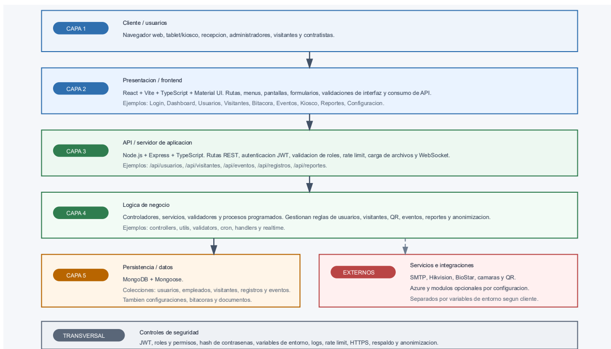
Ilustración 8. Arquitectura del sistema (separación de capas)
